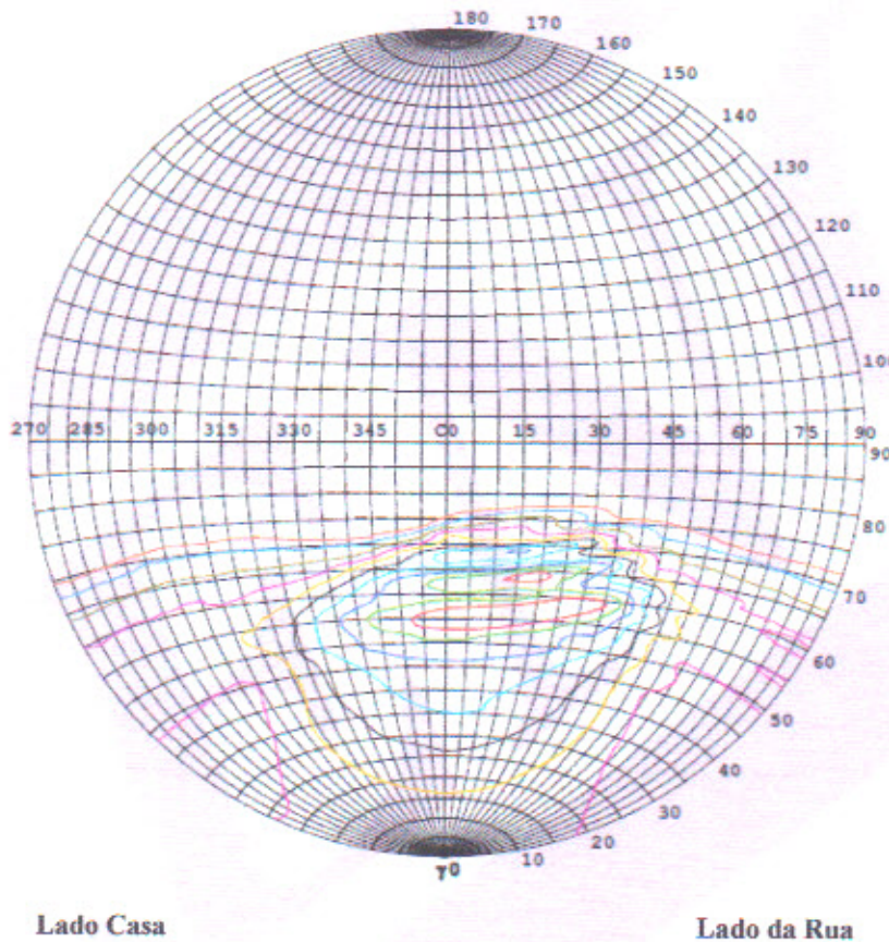
Figura 03 - Diagrama de Luz de Rua Isocandela
